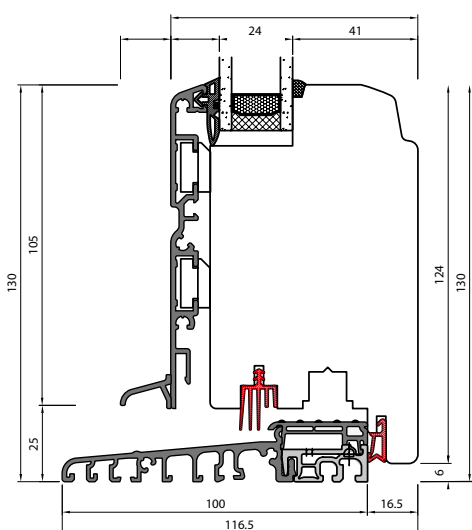
IDEALU CLASSICLINE IV 68 PORTE-FENÊTRE AVEC SEUIL PLAT
