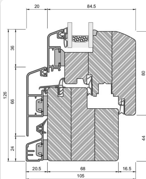
IDEALU CLASSICLINE IV 68 CHÂSSIS AVEC VANTAIL
