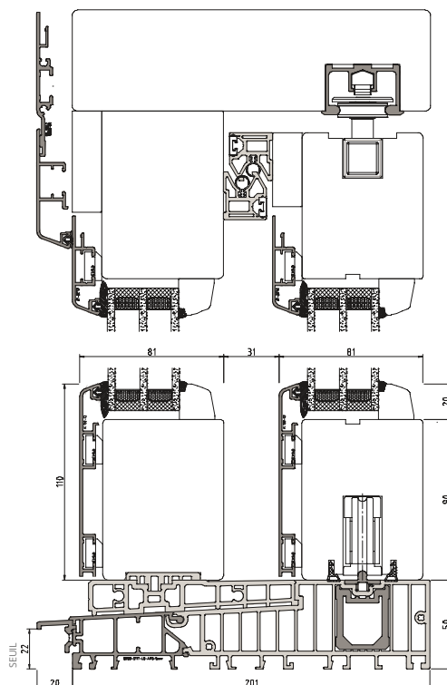
COUPE VERTICALE BAIE SOULEVANTE-COULISSANTE BOIS-ALU IDEALU IV 68
