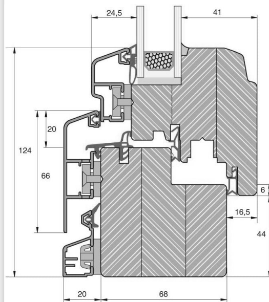
IDEALU TRENDLINE IV 68 CHÂSSIS AVEC VANTAIL
