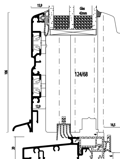
IDEALU TRENDLINE IV 68 AVEC SEUIL PLAT
