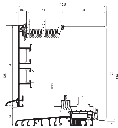
PORTE-FENÊTRE IDEAL PLANO AVEC SEUIL PLAT
