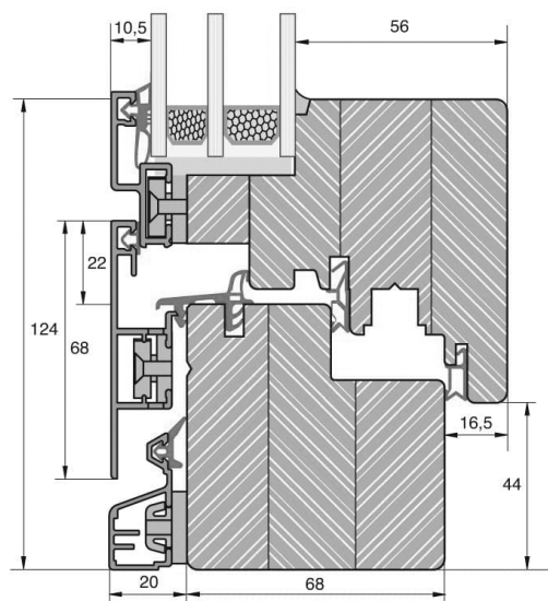
CHÂSSIS AVEC VANTAIL IDEAL PLANO
