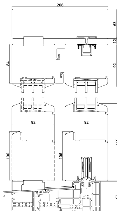
BAIE SOULEVANTE-COULISSANTE CLASSIQUE VI 92
