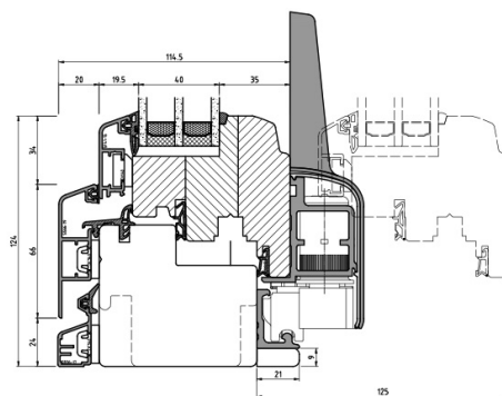
BAIE OSCILLO-COULISSANTE BOIS-ALU IDEALU CLASSICLINE IV 78
