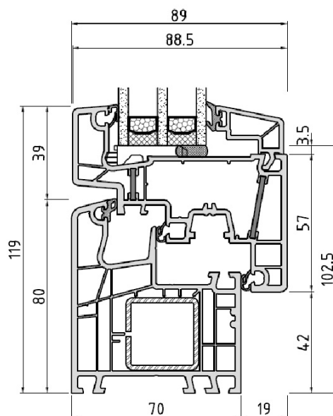
PROFILÉ IDEAL® DESIGN CADRE ET VANTAIL
