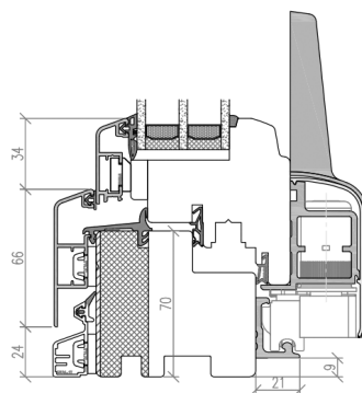
BAIE OSCILLO-COULISSANTE BOIS-ALU ECO IDEALU CLASSICLINE
