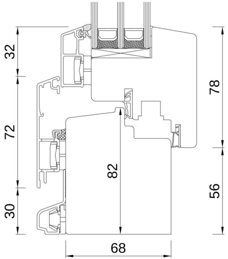
IDEALU Classicline IV 68 CHÂSSIS AVEC VANTAIL
