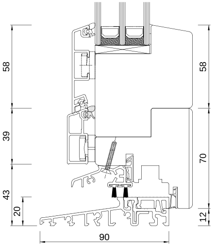
IDEALU Classicline IV 68 PORTE-FÊTÊTRE AVEC SEUIL PLAT
