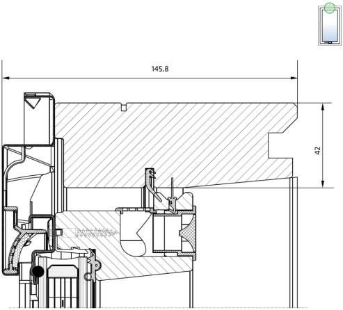
VUE DE DESSUS: OUVERTURE PAR ROTATION, DOUBLE VITRAGE
